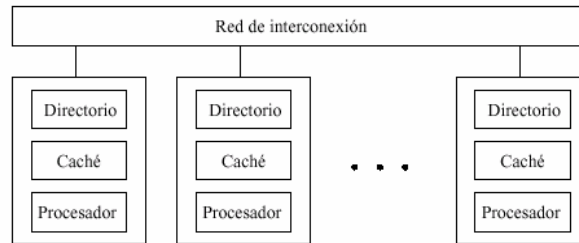
Figura 12: Ejemplo de COMA
