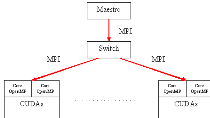
Figura 16: Paralelización Híbrida
