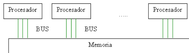
Figura 9: Arquitectura de una computadora paralela con memoria compartida
