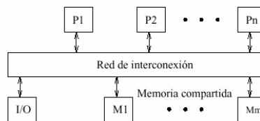
Figura 6: Acceso Uniforme a la memoria UMA
