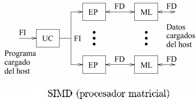
Figura 4: Ejemplo de máquina SIMD
