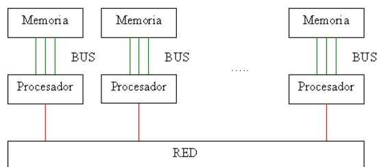
Figura 11: Arquitectura de una computadora paralela con memoria distribuida
