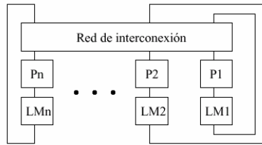
Figura 9: Acceso no uniforme a la memoria NUMA
