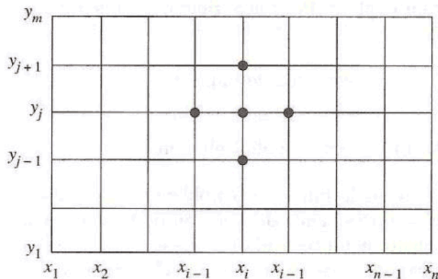
Figura 2: Discretización en un rectángulo.
