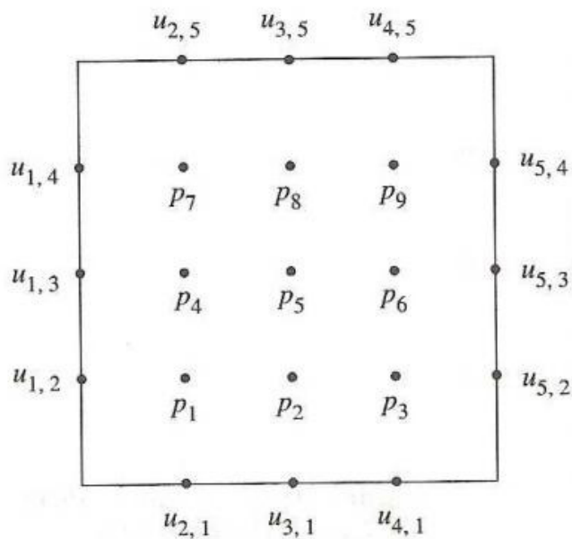
Figura 1: Si suponemos una malla discretizada en 5 \times 5 nodos, donde 9 serían interiores y 16 de frontera para tener un total de 25 nodos, donde la evaluación de los 9 nodos interiores los denotamos con p_1, \dots, p_9 .
