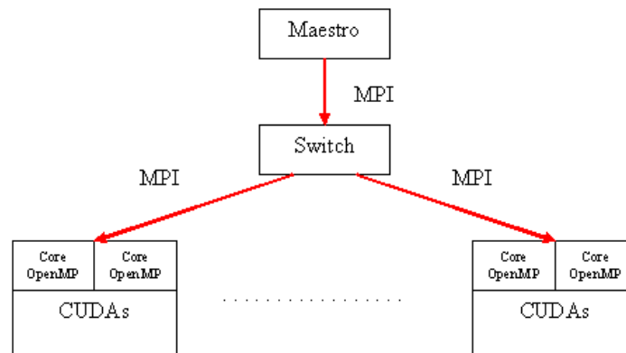
Figura 14: Paralelización Híbrida
