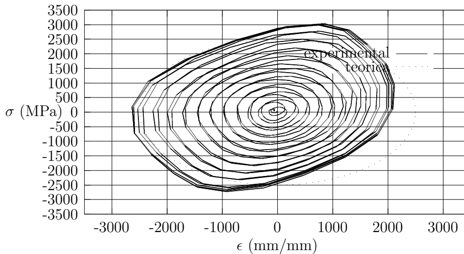
Carga fuera de fase para el acero 1045
