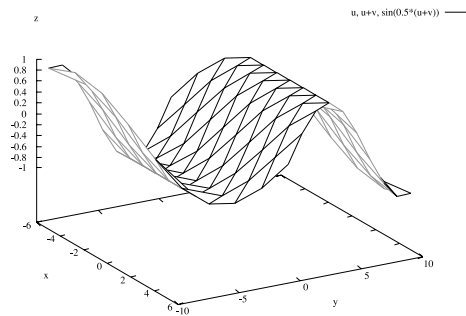
Fig. 16. ... set hidden3d ...
