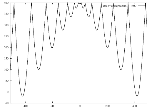
Fig. 20. plot [-512:512] -abs(x*sin(sqrt(abs(x))))+400
