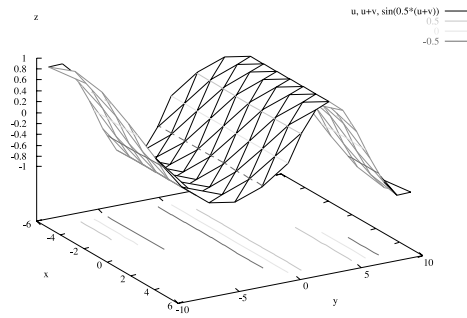
Fig. 17. ... set hidden3d ...
