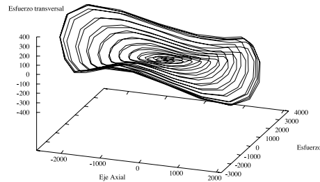
Fig. 18. ... set hidden3d ...
