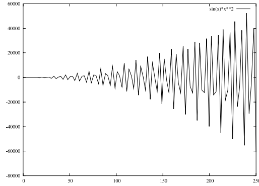
Fig. 5. plot sin(x)*(x**2)
