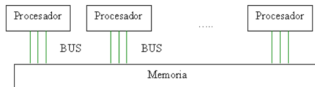
Figura 6: Arquitectura de una computadora paralela con memoria compartida
