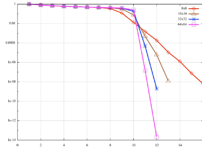
Figura 17: Residual relativo para la malla local de 16 \times 16 , en este caso \underline{b} = (1, 3) y \nu = 0.00001 que corresponde a un valor de Pe = 3.16e + 5 .
