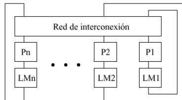
Figura 8: Acceso no uniforme a la memoria NUMA
